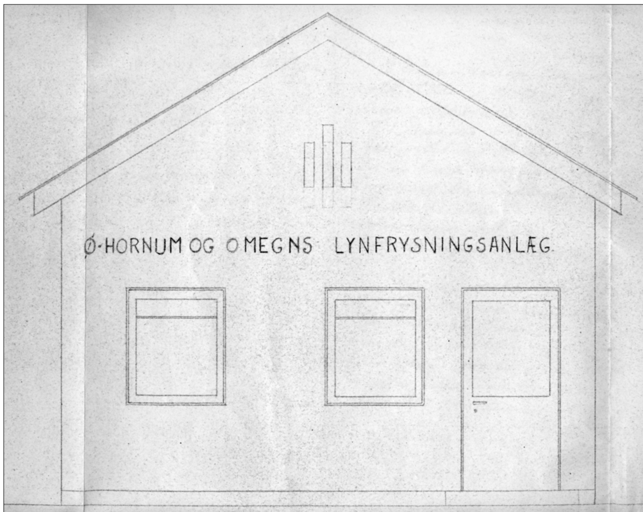
Tegning af Ø. Hornum og Omegns Lynfrysningssanlægs facade ud mod Nihøjevej, udarbejdet af Lindholm og Ryø, Aalborg 24. august 1950
