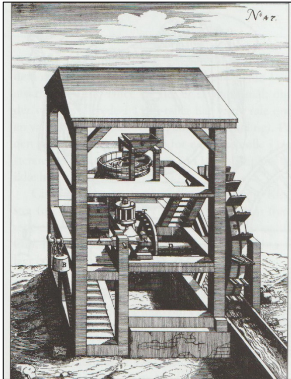
Padlebladsmølle efter Georg A. Böcklern, Theatrum Machinarum Novum, Nürnberg 1661. Jf. Lise Andersen, Træk af dansk møllebyggeris historie, s. 17.
